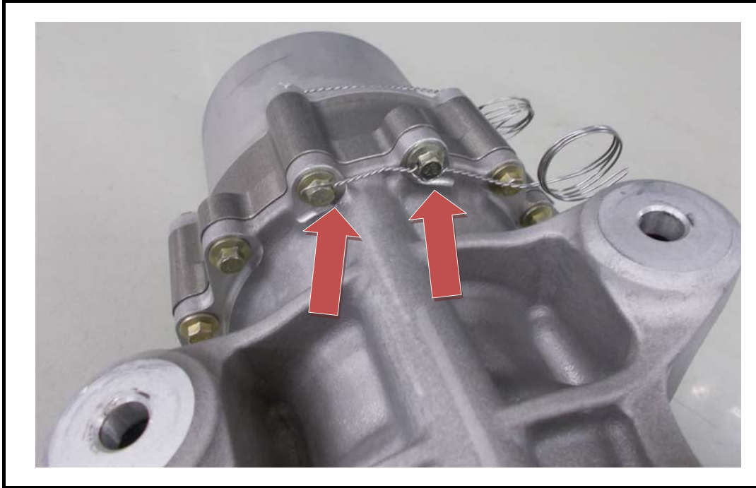
A) SEAL n°1
